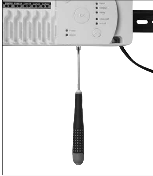
Adım 4) DIN rayından demontaj
