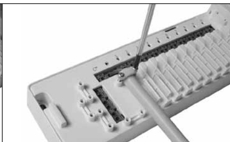
Adım 6) Sirkülasyon pompasının kontrol edilebilmesi için kablonun bağlanması.
